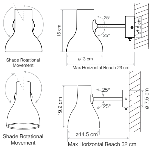
Type 75™ Mini Wall Light
